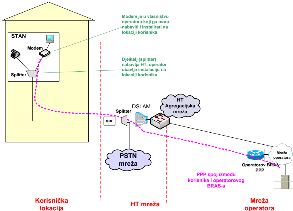
Slika 9. Način realizacije Veleprodajnog širokopojsnog pristupa za pružanje Internet usluge na DSLAM razini
