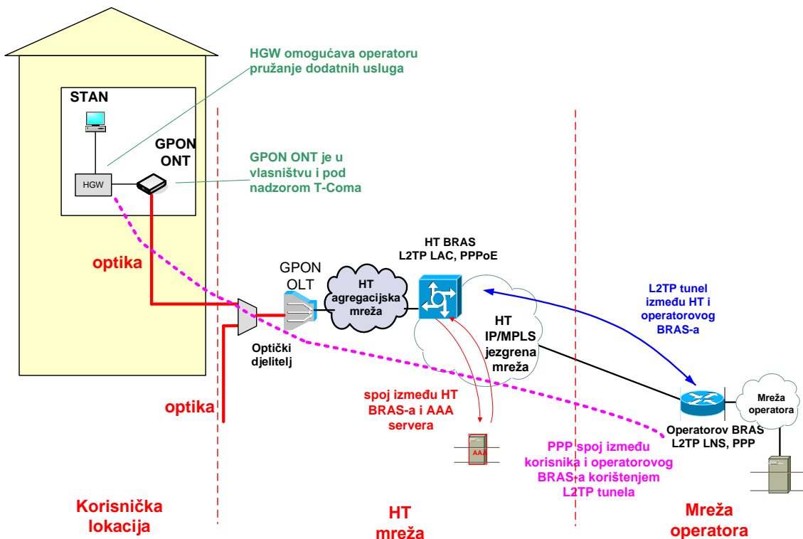
Slika 2. Način realizacije usluge veleprodajnog širokopojsnog pristupa za Internet uslugu na temelju FTTH rješenja na IP razini
