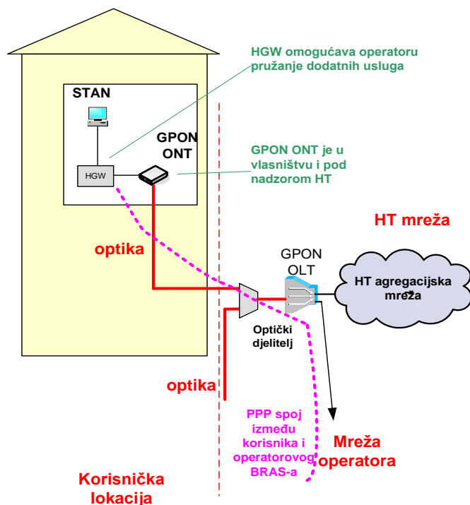
Slika 6. Način realizacije usluge veleprodajnog širokopojasnog pristupa za Internet uslugu na temelju FTTH rješenja na OLT razini
