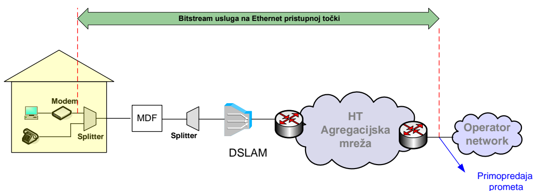
Slika 3. Veleprodajni širokopolasni pristup za pružanje Internet usluge na Ethernet razini u slučaju kada Krajnji korisnik ostvaruje Osnovni pristup mreži putem usluge HT-a.
